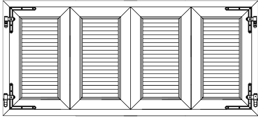
DIŞTAN GÖRÜNÜŞ
