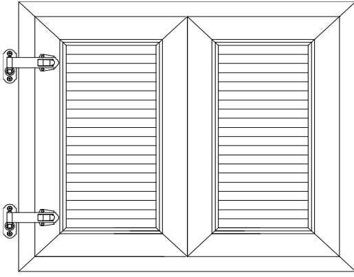
DIŞTAN GÖRÜNÜŞ
