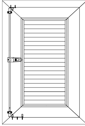
İÇTEN GÖRÜNÜŞ
