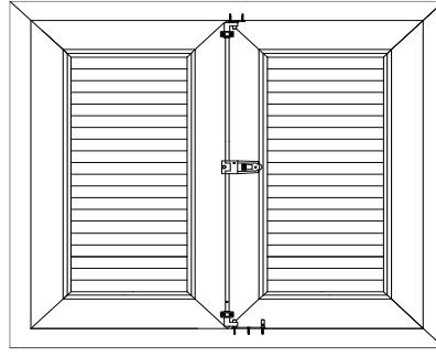
İÇTEN GÖRÜNÜŞ
