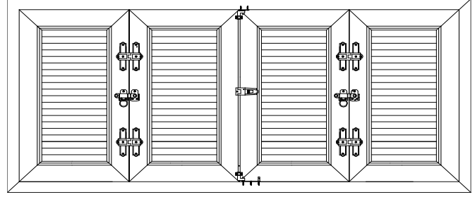
İÇTEN GÖRÜNÜŞ
