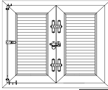
İÇTEN GÖRÜNÜŞ
